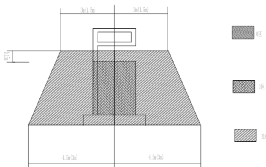
图 3-1 加油机爆炸危险区域划分
