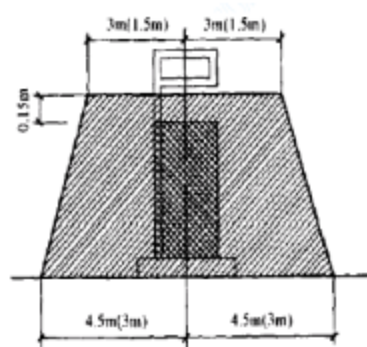
图 3.2-2 汽油加油机操作危险区域划分图
