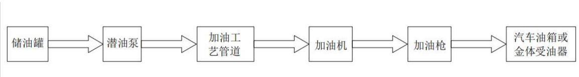
图 2-4 柴油加油工艺框图
