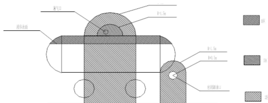
图 3-1 加油机爆炸危险区域划分
