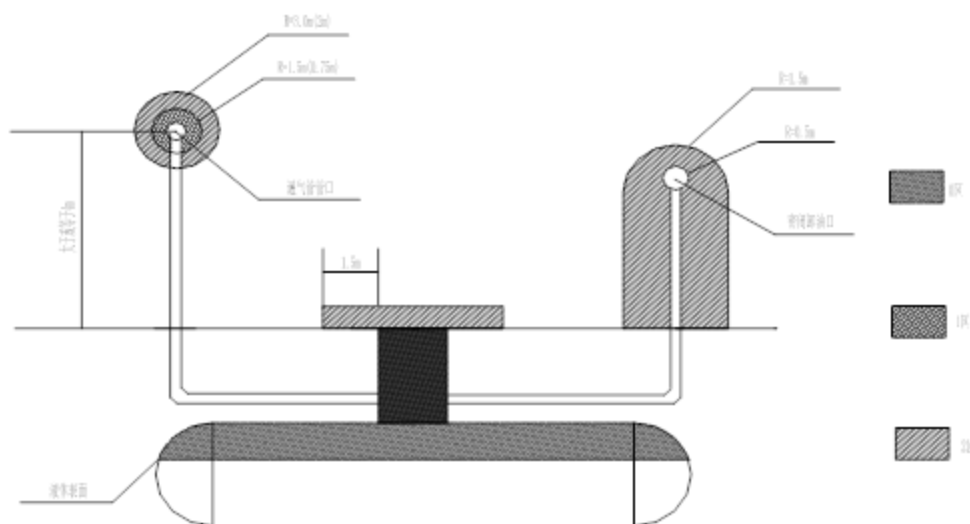
图 3-2 油罐车卸油爆炸危险区域划分
