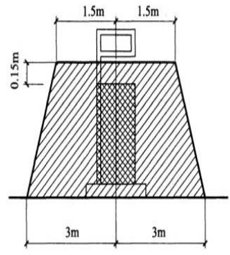
图 2-2 加油机操作危险区域划分
