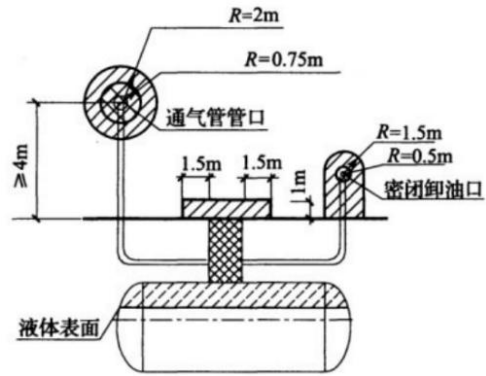
图 2-1 埋地卧式储罐爆炸危险区域划分
