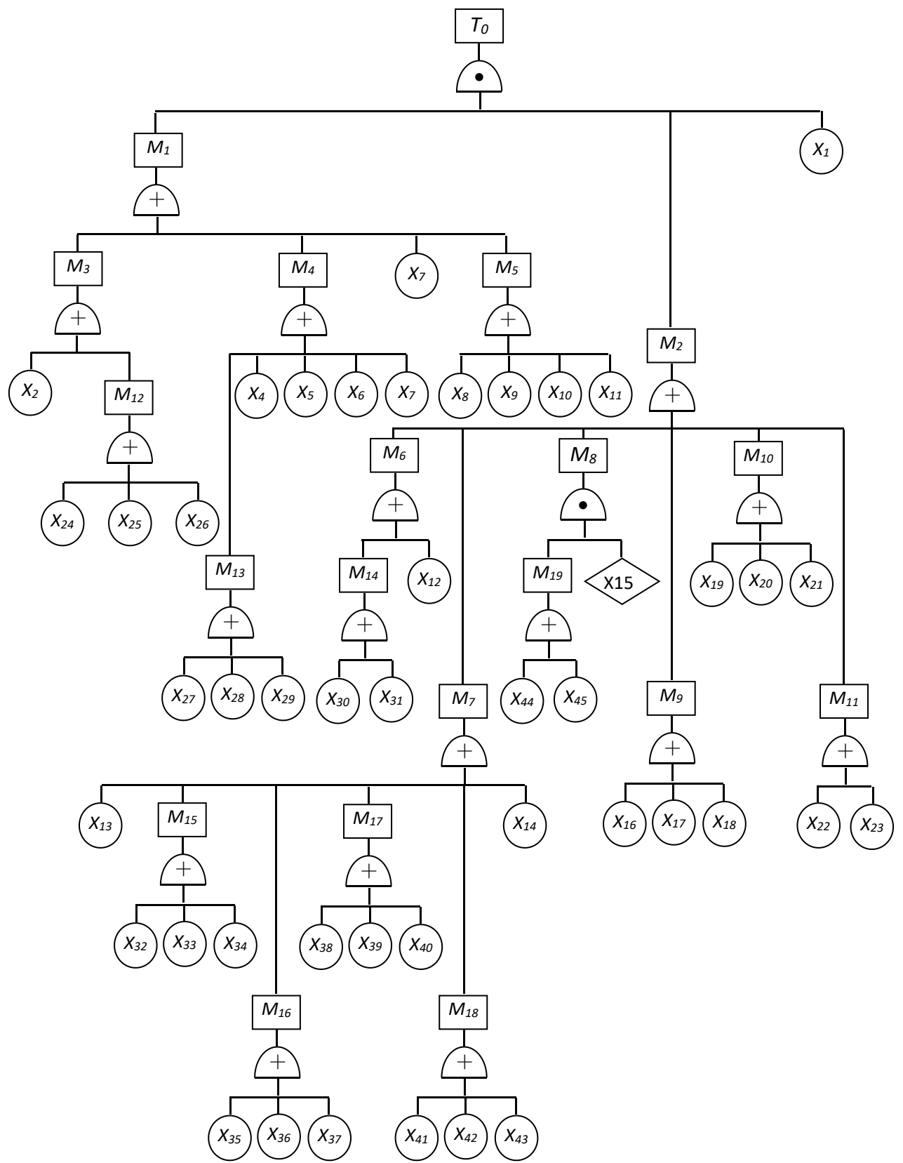
图 F2.2-1 事故树分析
